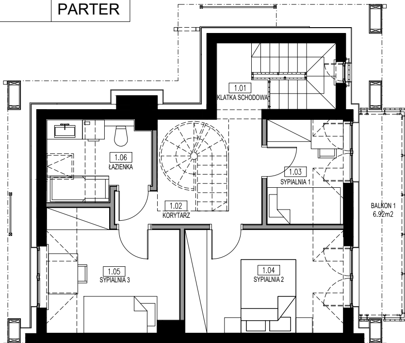
PIĘTRO I
